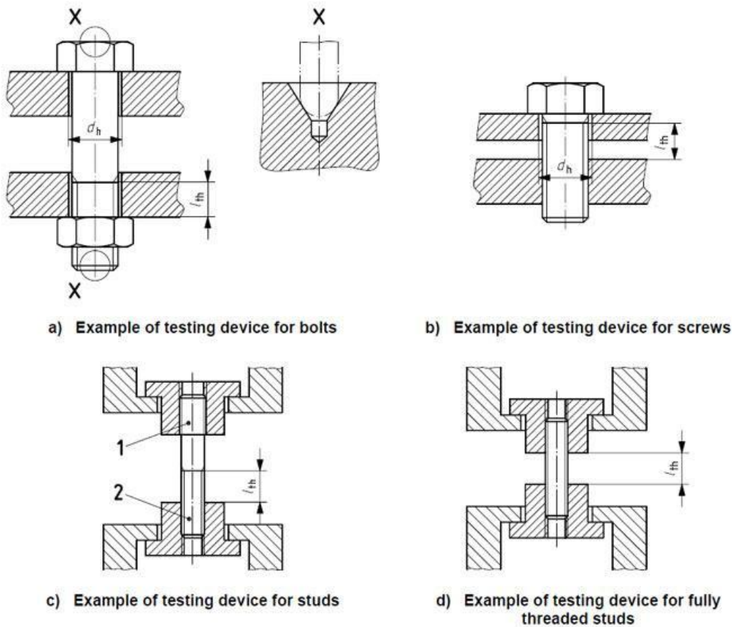
紧固件成品施加保证载荷安装示例
