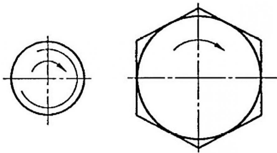
左旋螺纹的螺栓和螺钉的标志
