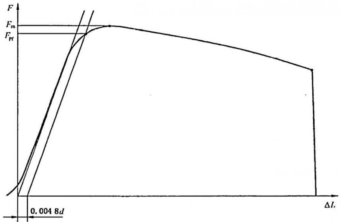
测定 0.0048d 非比例延伸应力 R Pf 的载荷-位移曲线
