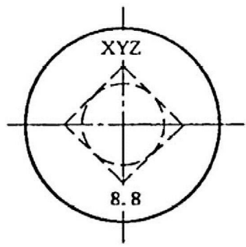
圆头方颈螺栓标志示例
